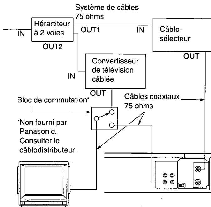
Vers l'entrée VHF 75 ohms du téléviseur
